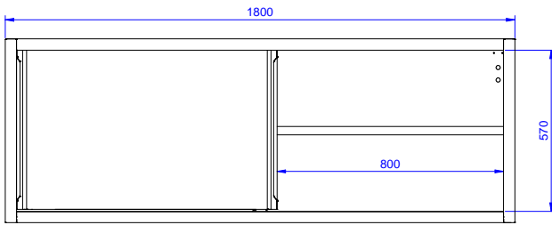
Front aanzicht
